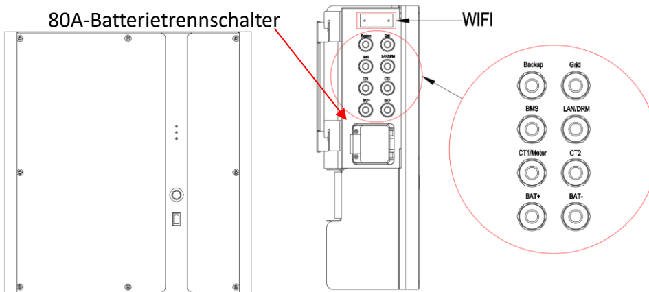
Abbildung 3. SMILE-B3 Systembeschreibung – linke Seite – Anschlüsse
