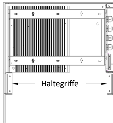
Abbildung 4. SMILE-B3 Systembeschreibung – Rückseite – Haltegriffe
